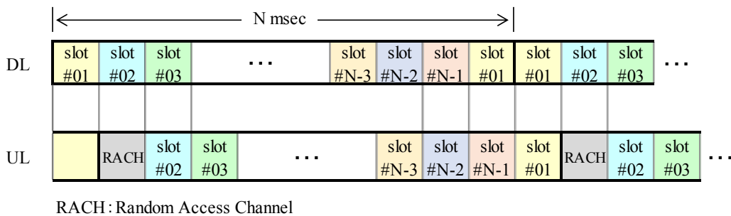
図 4.3 無線システムにおけるフレーム構成
