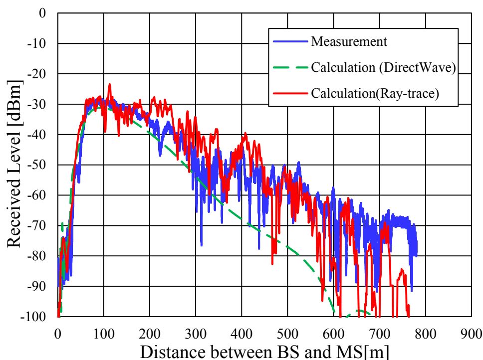
図 3.10 レイトレース法の電界強度シミュレーション結果と実測値の比較 ( R=2500\text{m} 防音壁無)
