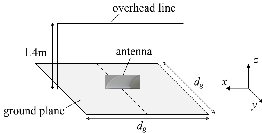
図 2.19 試作アンテナ測定時の地板，架線の条件
