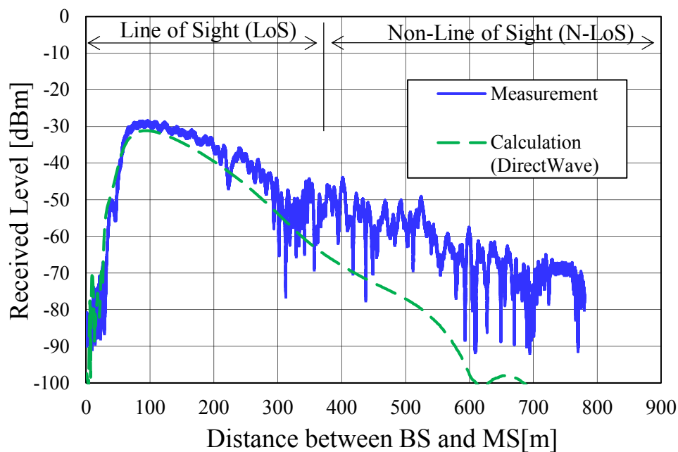
図 3.8 R=2500\text{m} 曲線区間（防音壁無）の受信電力
