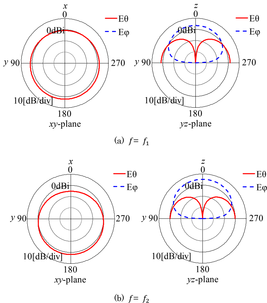
図 2.8 従来アンテナの放射パターン計算結果
