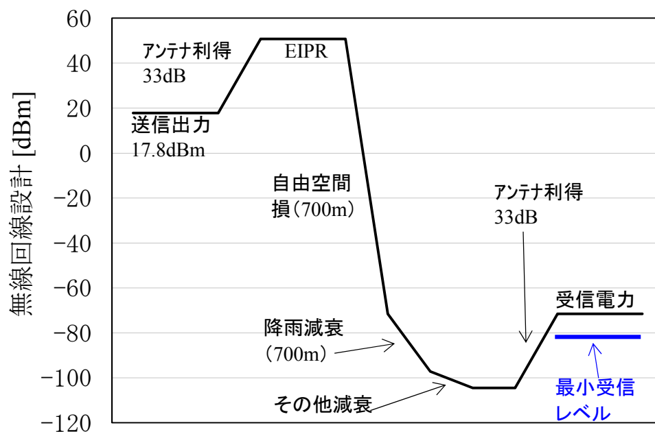
図 4.8 基本的な回線設計（地上局車上局間 700 m）
