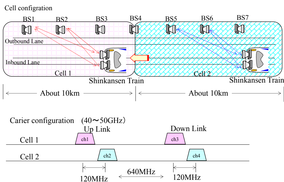
図 4.2 セルの構成とキャリア配置
