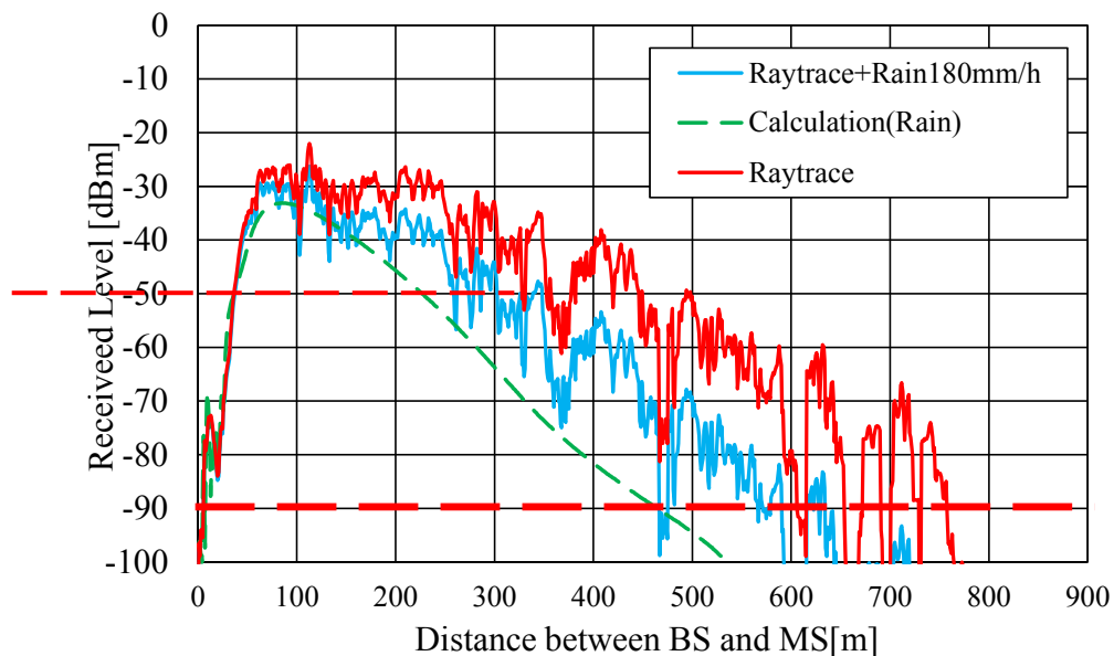
図 4.11 提案方式における回線設計を適用した受信信号レベル (曲線区間 R=2500 m, 防音壁無し)
