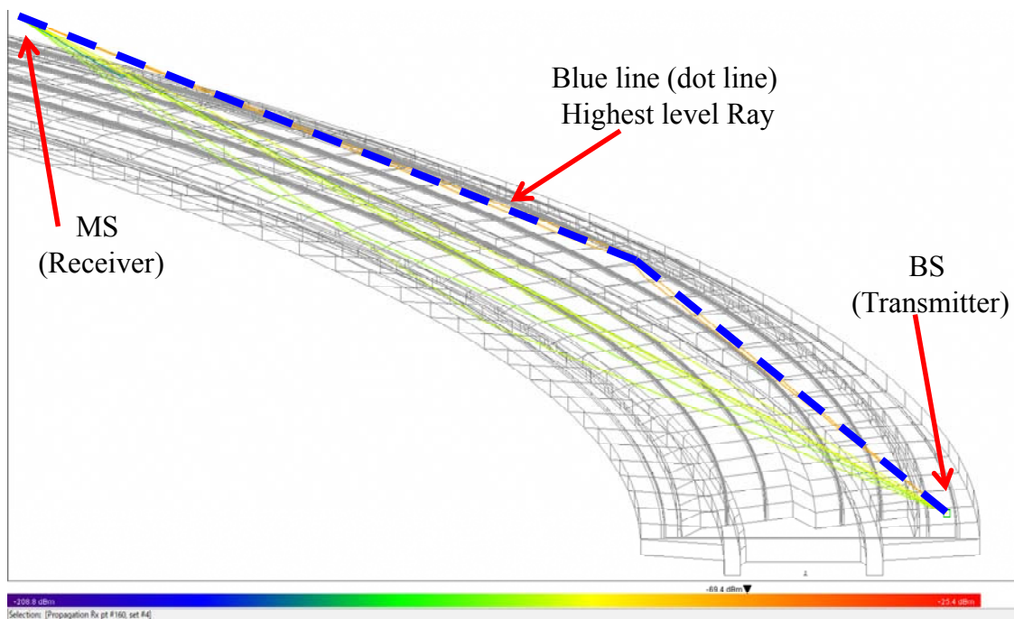
図 3.15 レイトレース法のシミュレーション結果 レイの表示 ( R = 395 m 防音壁無，地上局車上局間 150 m)
