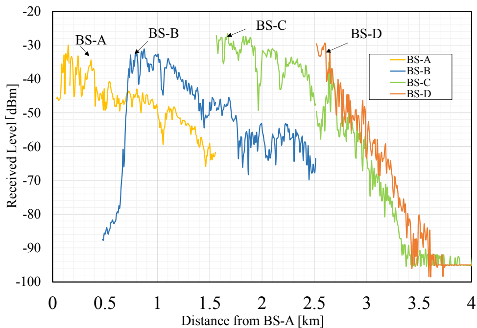
図 5.8 走行試験時の受信信号電力（セル内ハンドオーバ）
