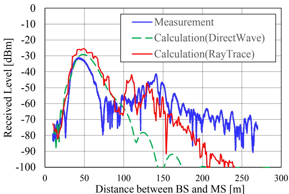
図 3.14 レイトレース法の電界強度シミュレーション結果と実測値の比較 ( R = 395\text{m} 防音壁無)
