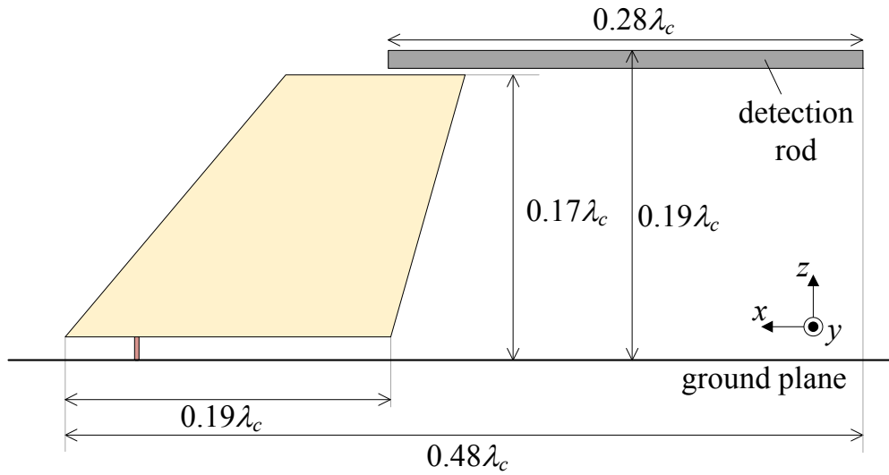
図 2.4 キャラクタリスティックモード解析における計算モデル
