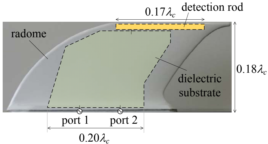
図 2.18 試作した提案アンテナ
