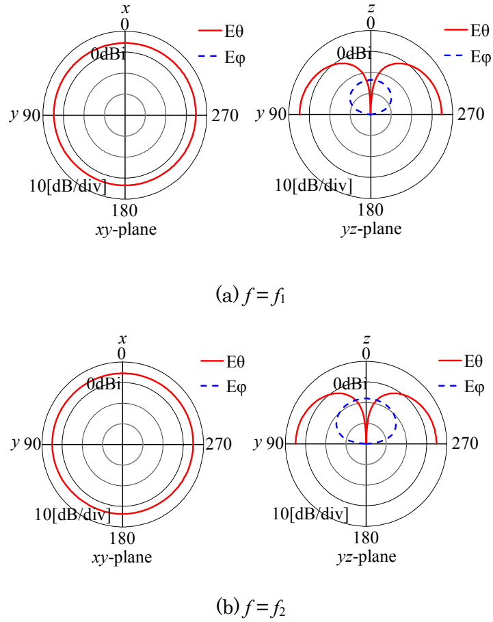
図 2.17 提案アンテナ (図 2.10) の放射パターン計算結果
