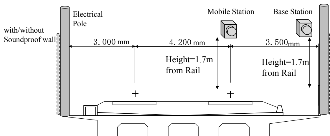
図 3.4 測定時の無線機設置条件
