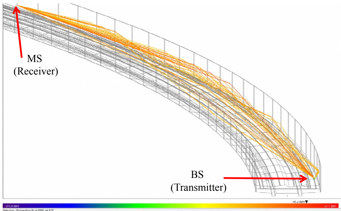
図 3.13 レイトレース法のシミュレーション結果 レイの表示 ( R = 2500 m 防音壁有, 地上局車上局間 500 m)
