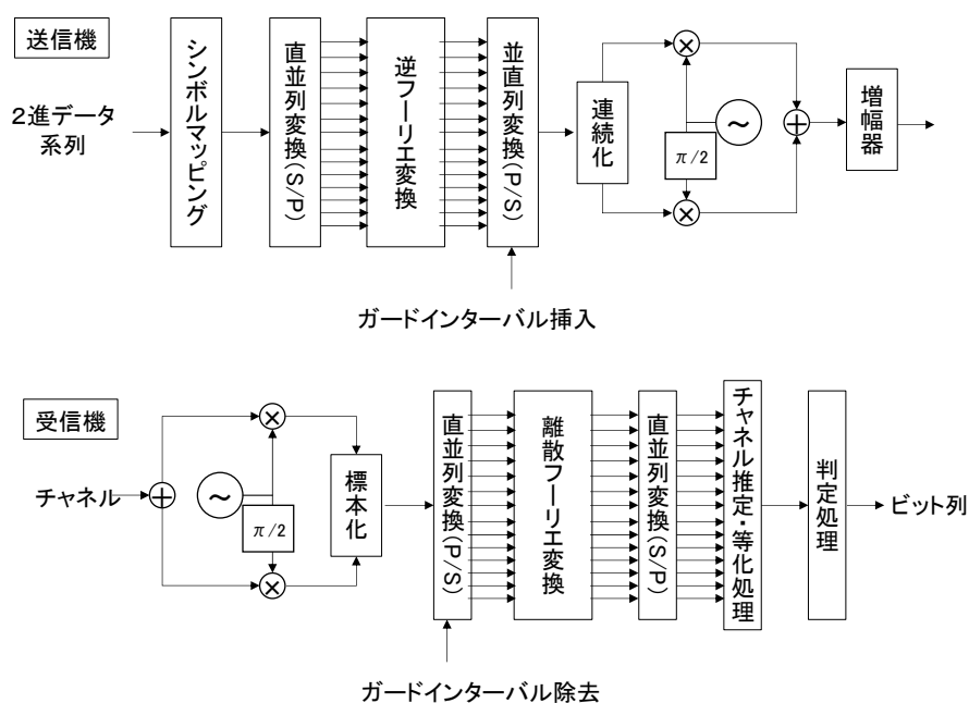
図 3.1 OFDM システムの送信機構成
