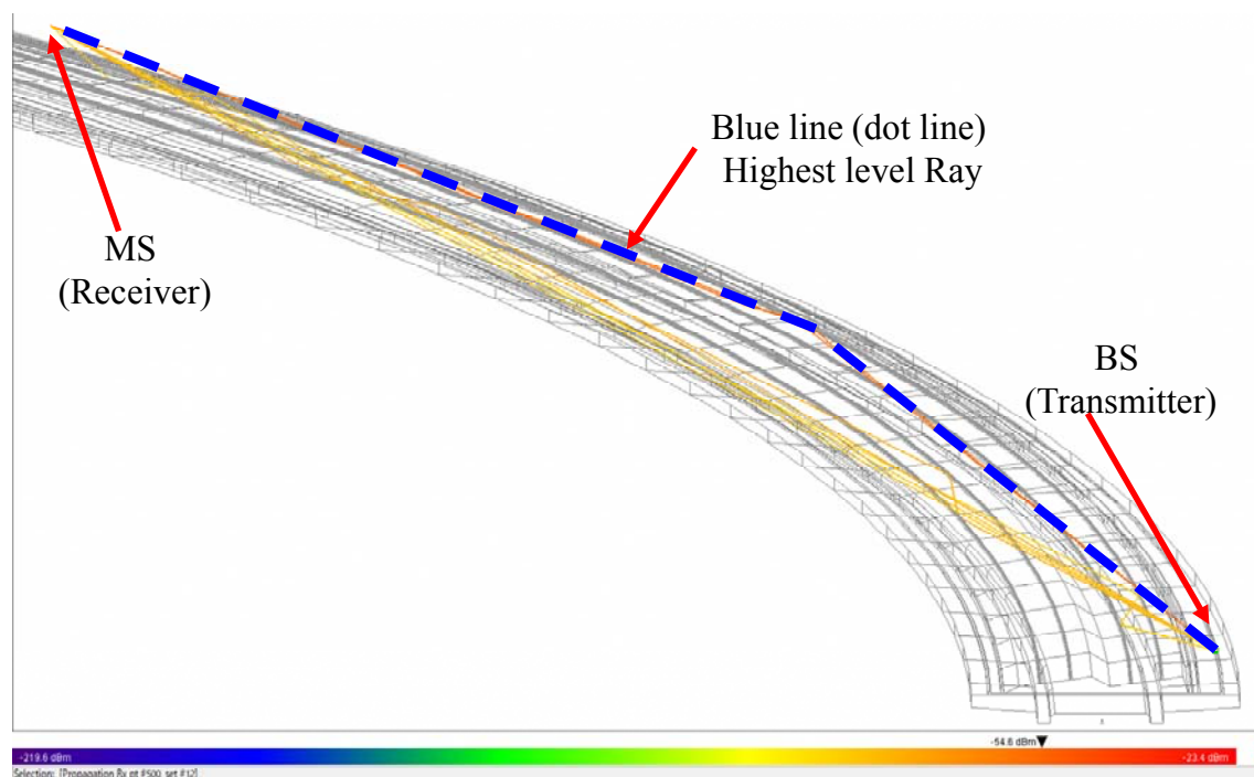
図 3.11 レイトレース法のシミュレーション結果 レイの表示 ( R = 2500 m 防音壁無，地上局車上局間 500 m)
